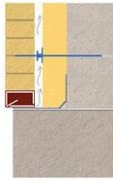
Разрез стены над фундаментом
