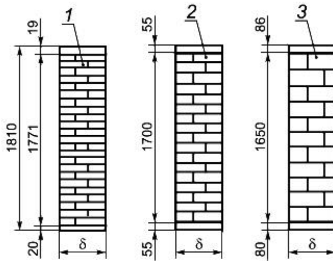
б) Примеры кладок в поперечном сечении
