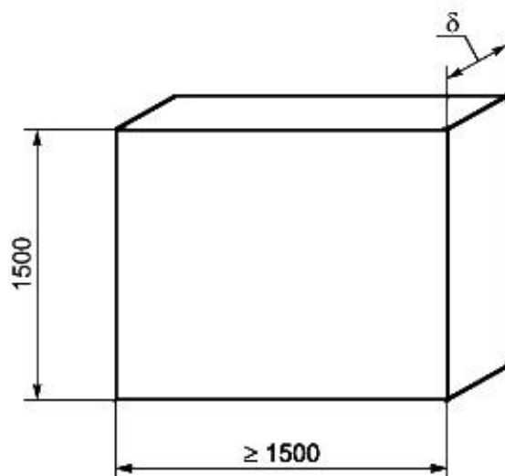
а) Общий вид кладки
